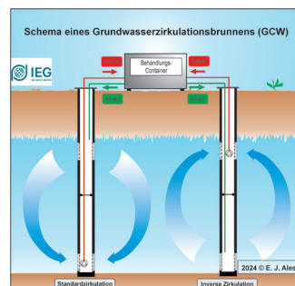
Abb. 1: Schema eines Grundwasserzirkulationsbrunnens im Standard-Zirkulationsmodus (SZ, links) und in inverser Zirkulation (IZ, rechts)
